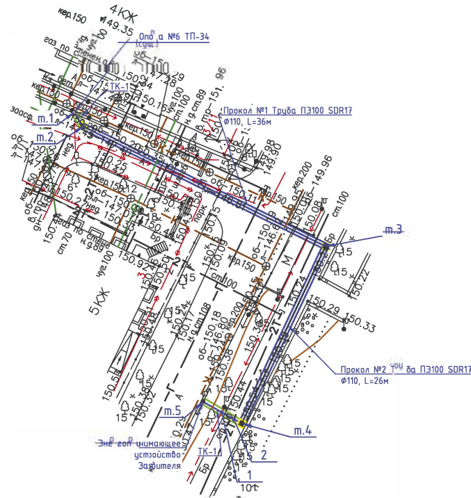
План трассы КЛ 0,4 кВ. М1:500
