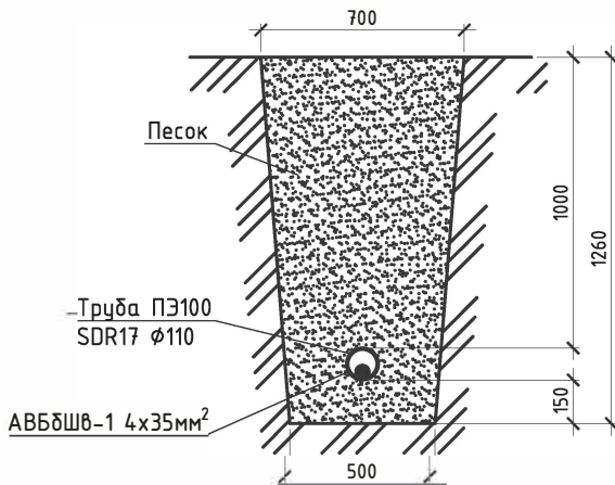
Разрез кабельной траншеи ТК-1
